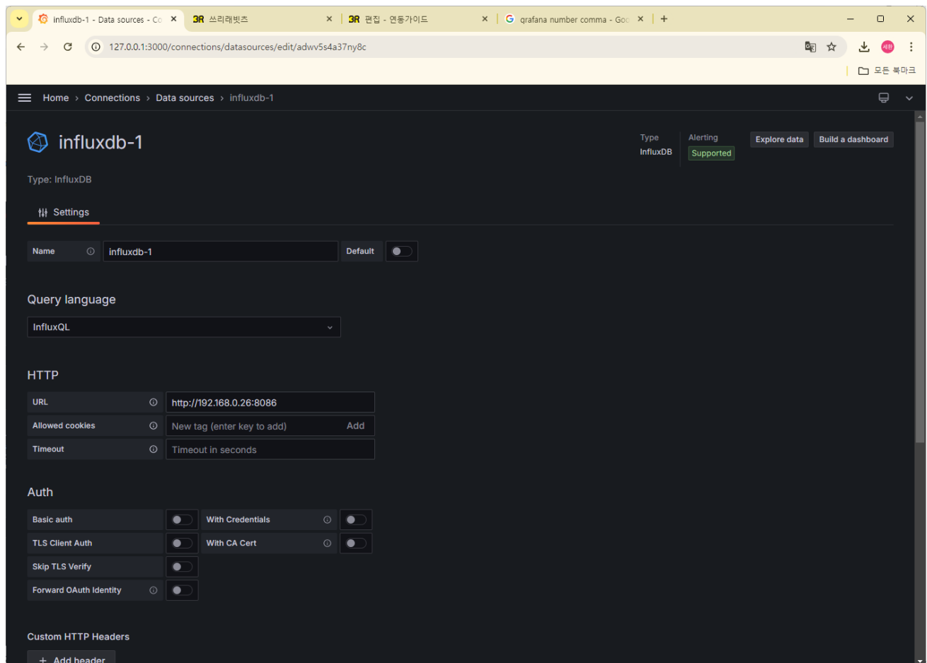
그림 7 Datasource
