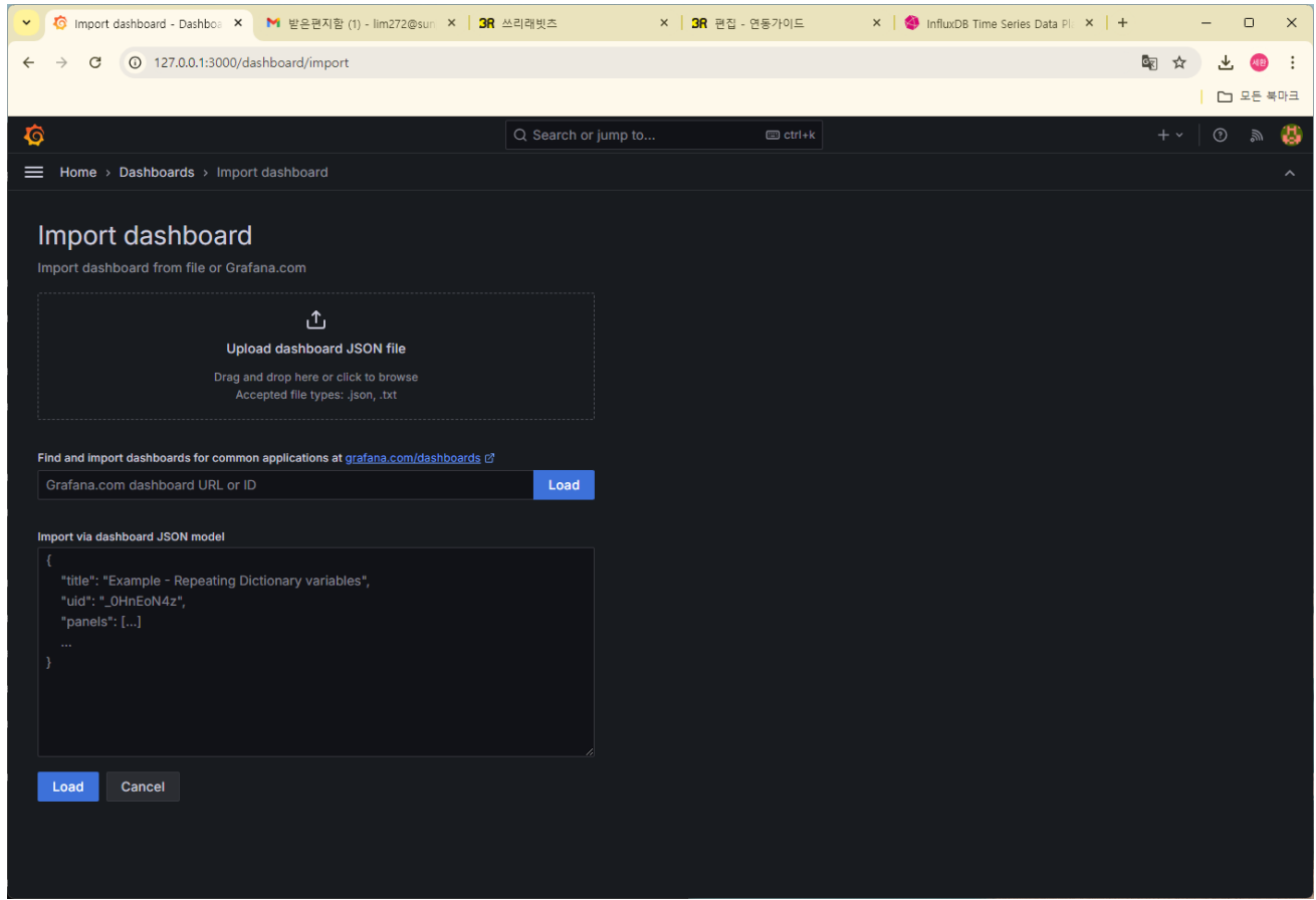
그림 9 Upload json
