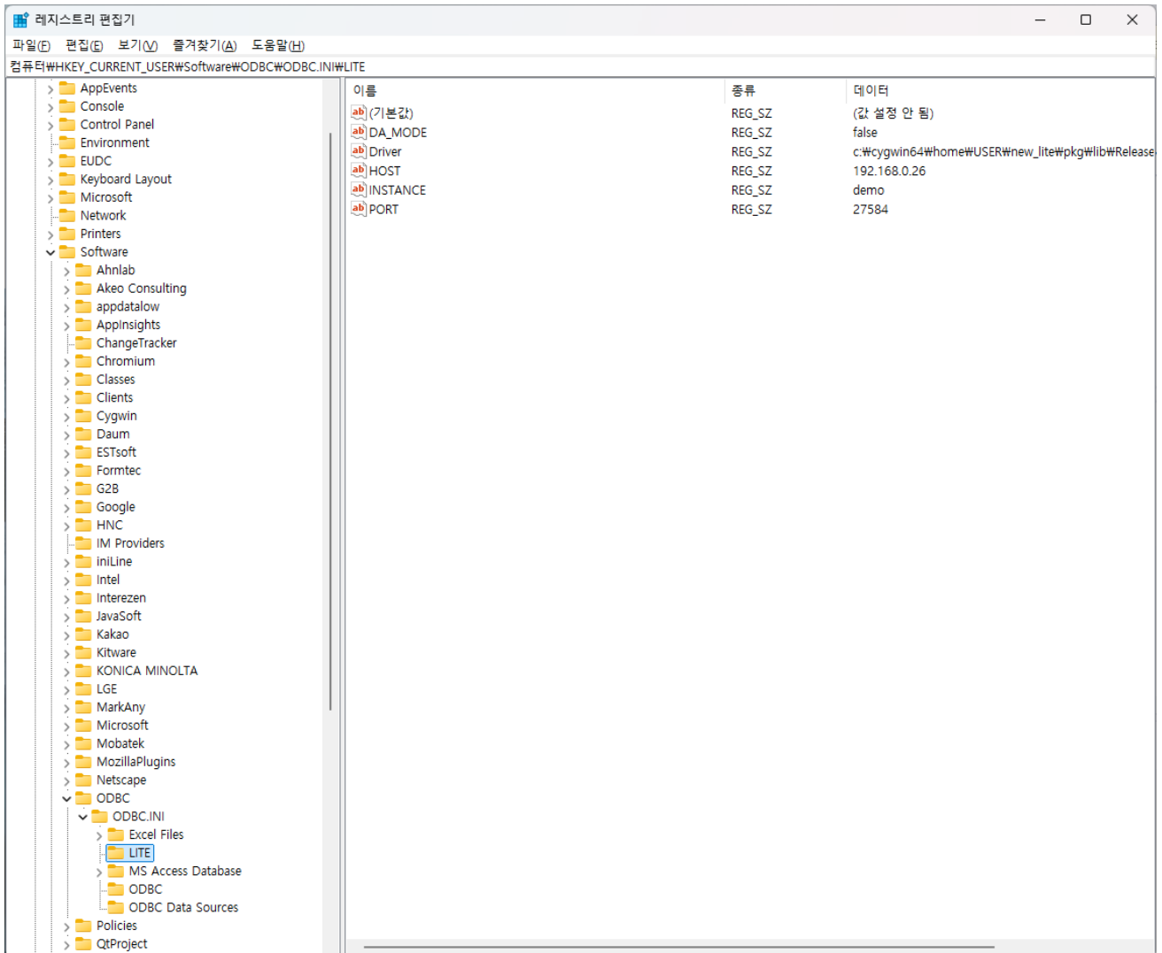
그림 6 DSN_sample
