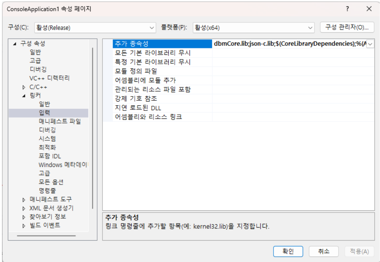
그림 5 library2
