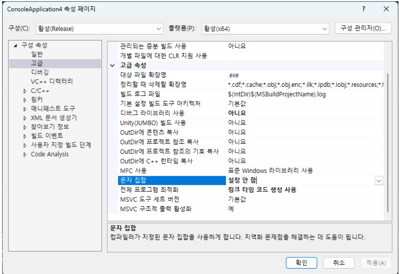
그림 2 문자 집합
