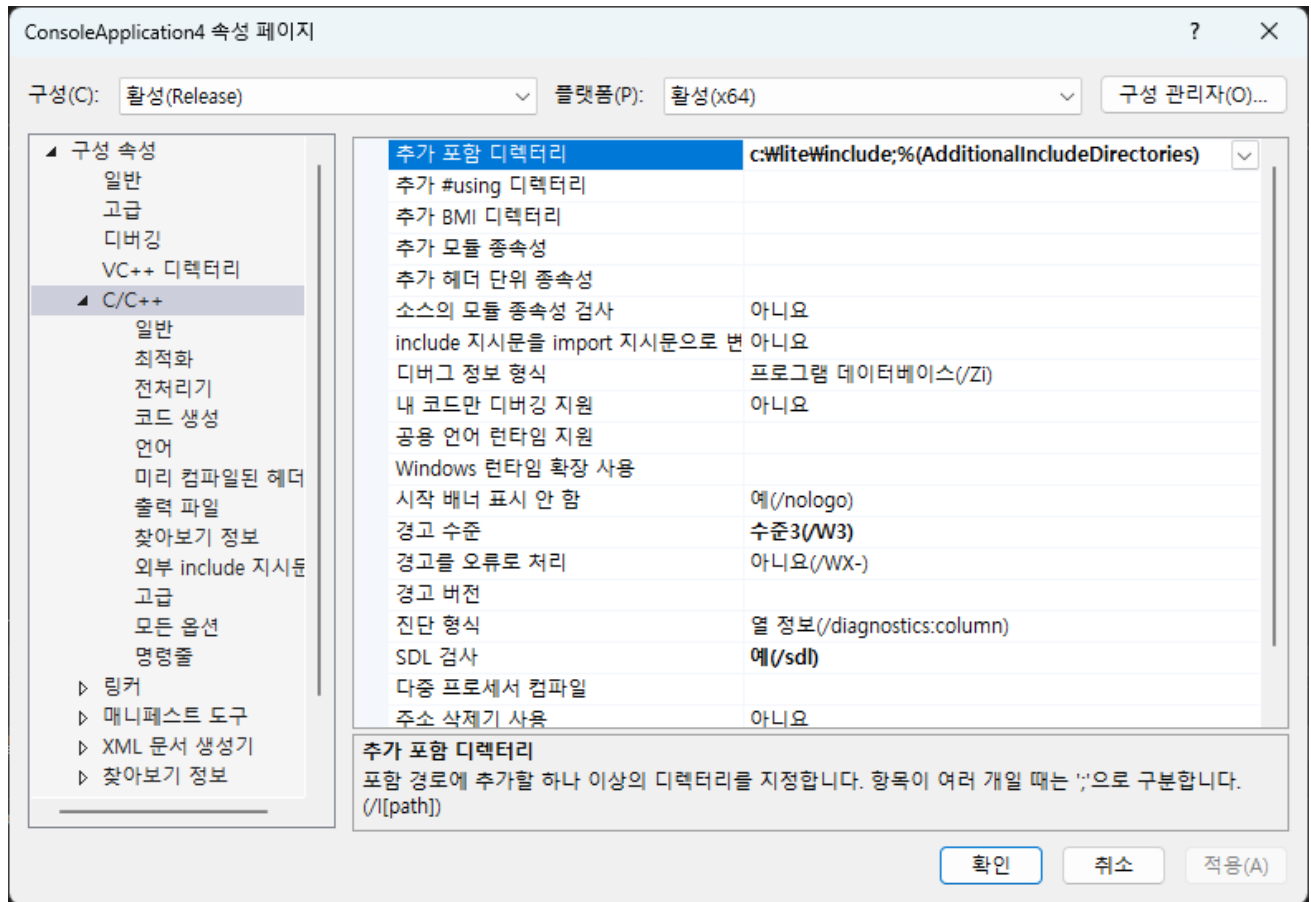
그림 3 헤더 경로
