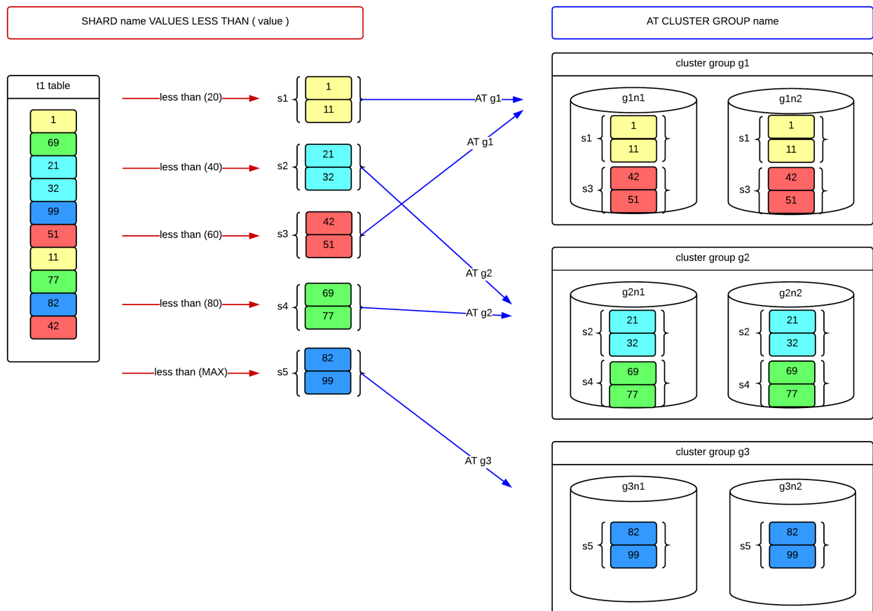
그림 10 Group-specific range-sharded table
