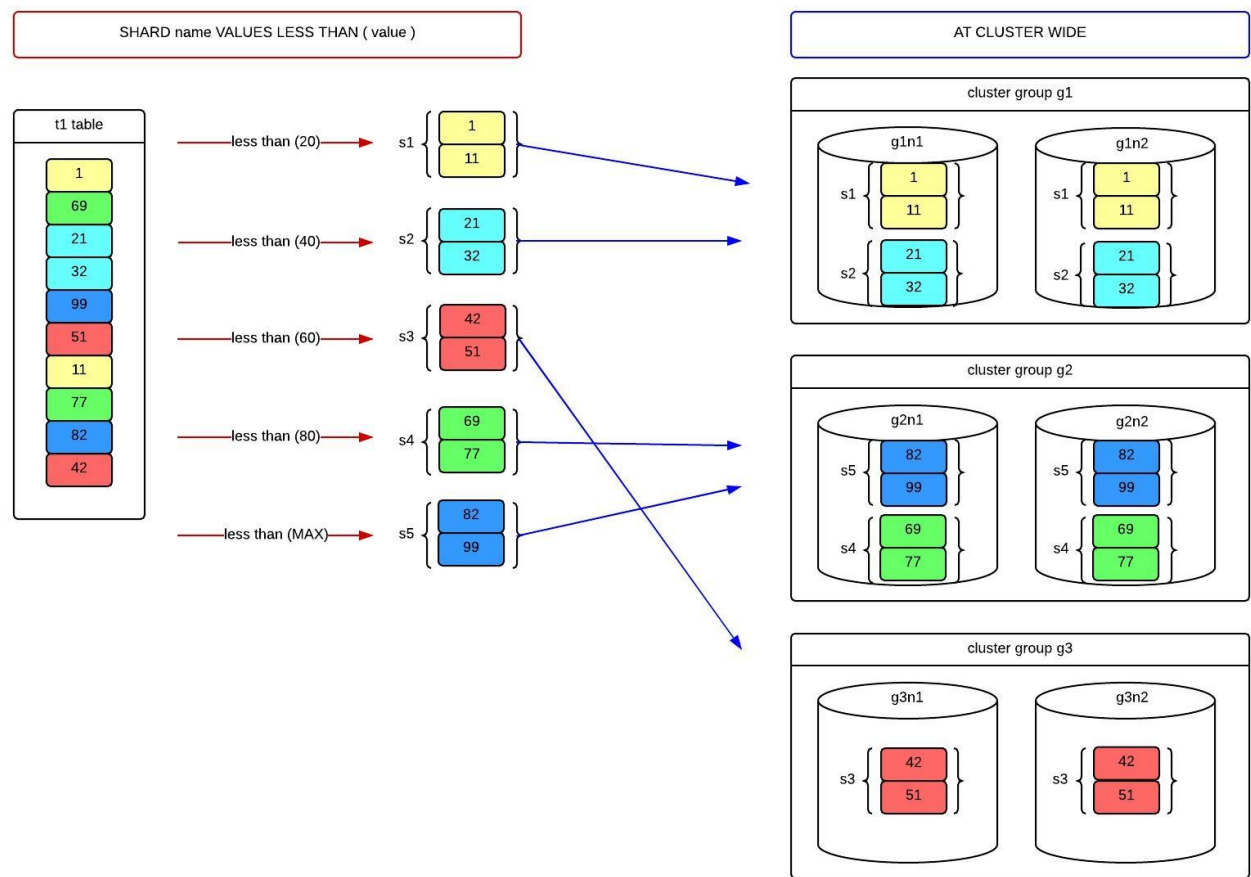
그림 9 Cluster-wide range-sharded table
