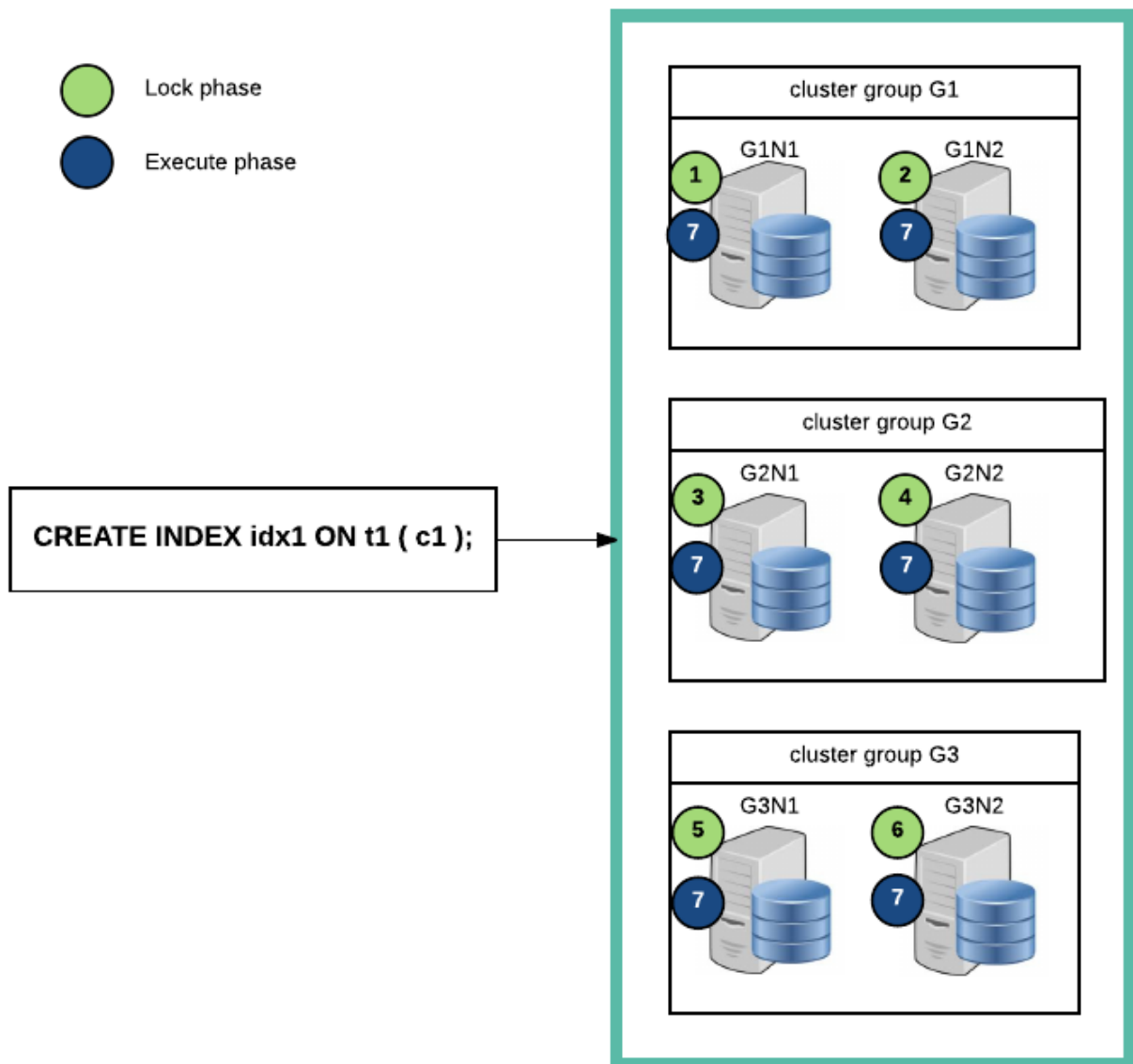
그림 1 Cluster의 DDL 처리 과정
