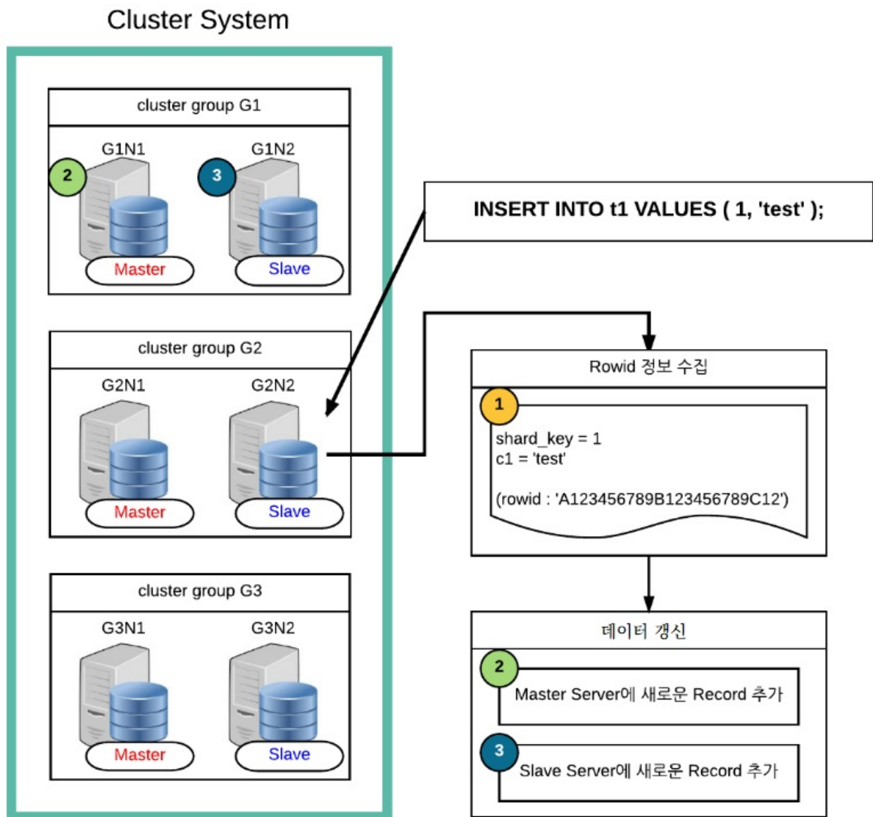
그림 6 Global secondary index를 사용하지 않는 rowid를 이용한 데이터 갱신
