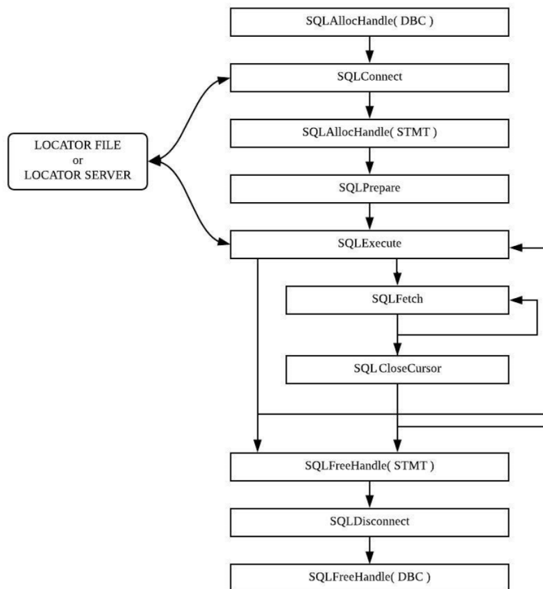
그림 7 Basic steps of applying GLOBAL CONNECTION
