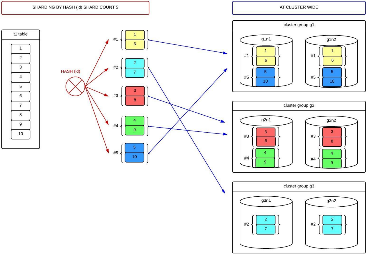
그림 7 Cluster-wide hash-sharded table
