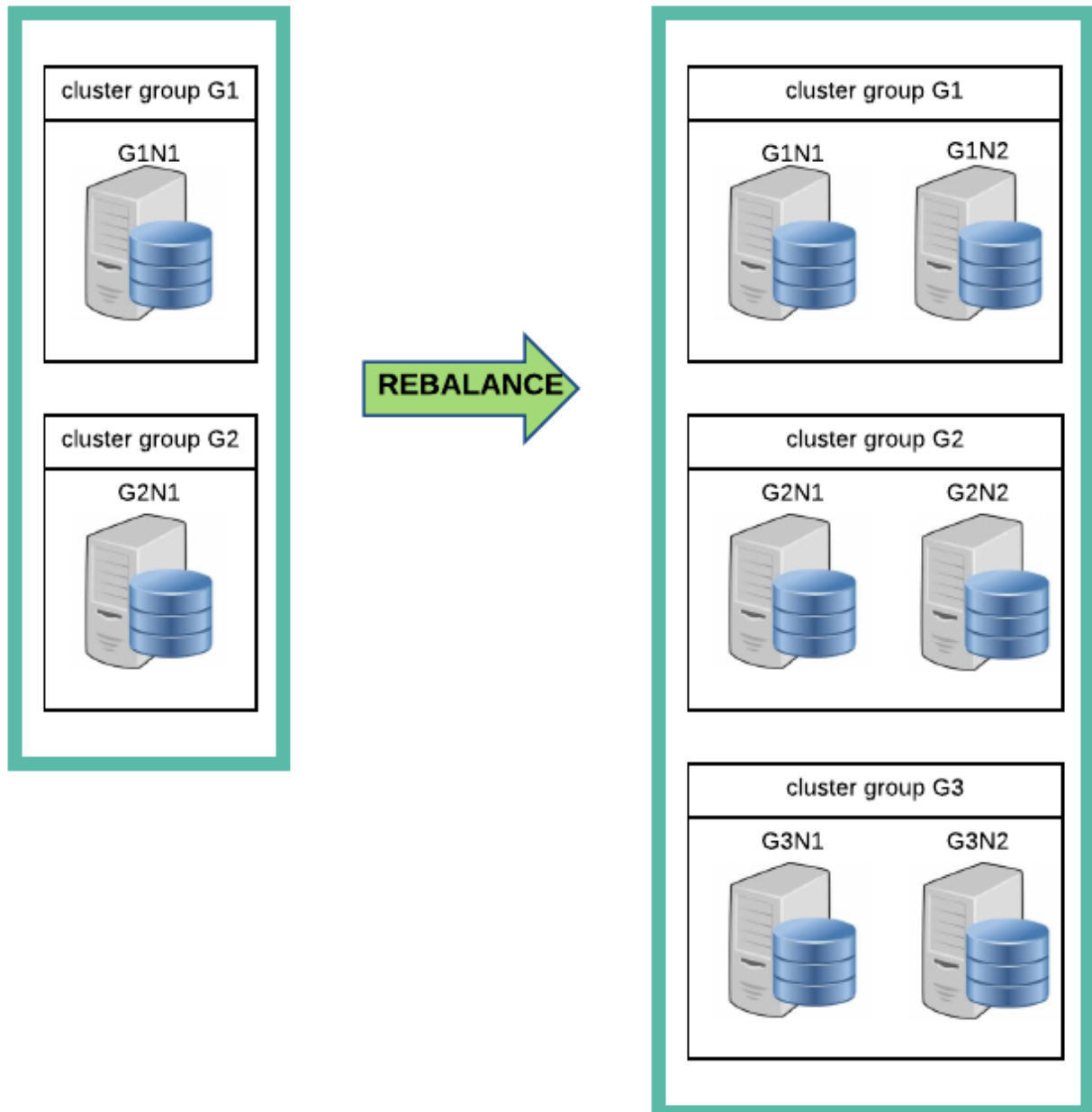
그림 13 AT CLUSTER WIDE로 정의한 region 테이블의 재배포
