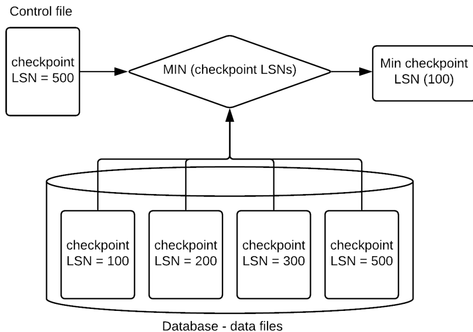
그림 2 Recovery를 위한 최소 checkpoint LSN을 구하는 과정
