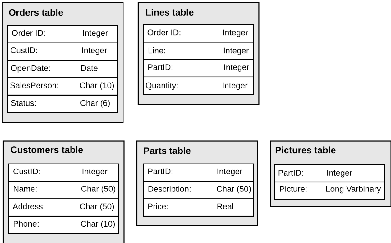
그림 8 Sales orders 구조체
