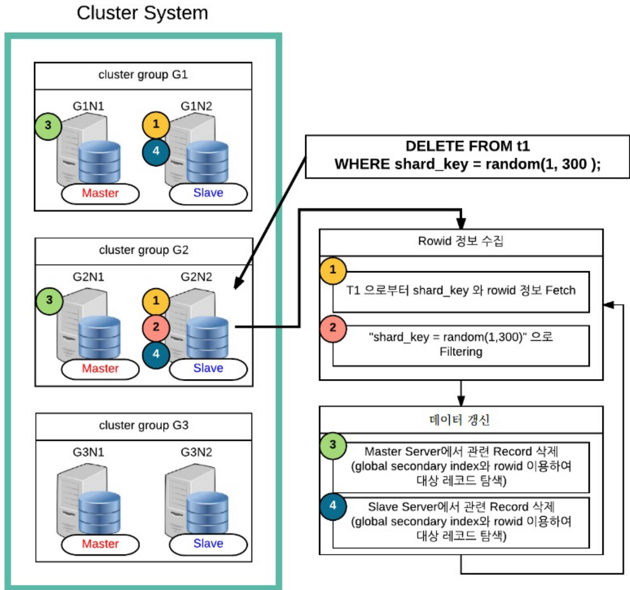
그림 7 Global secondary index를 사용하는 rowid를 이용한 데이터 갱신
