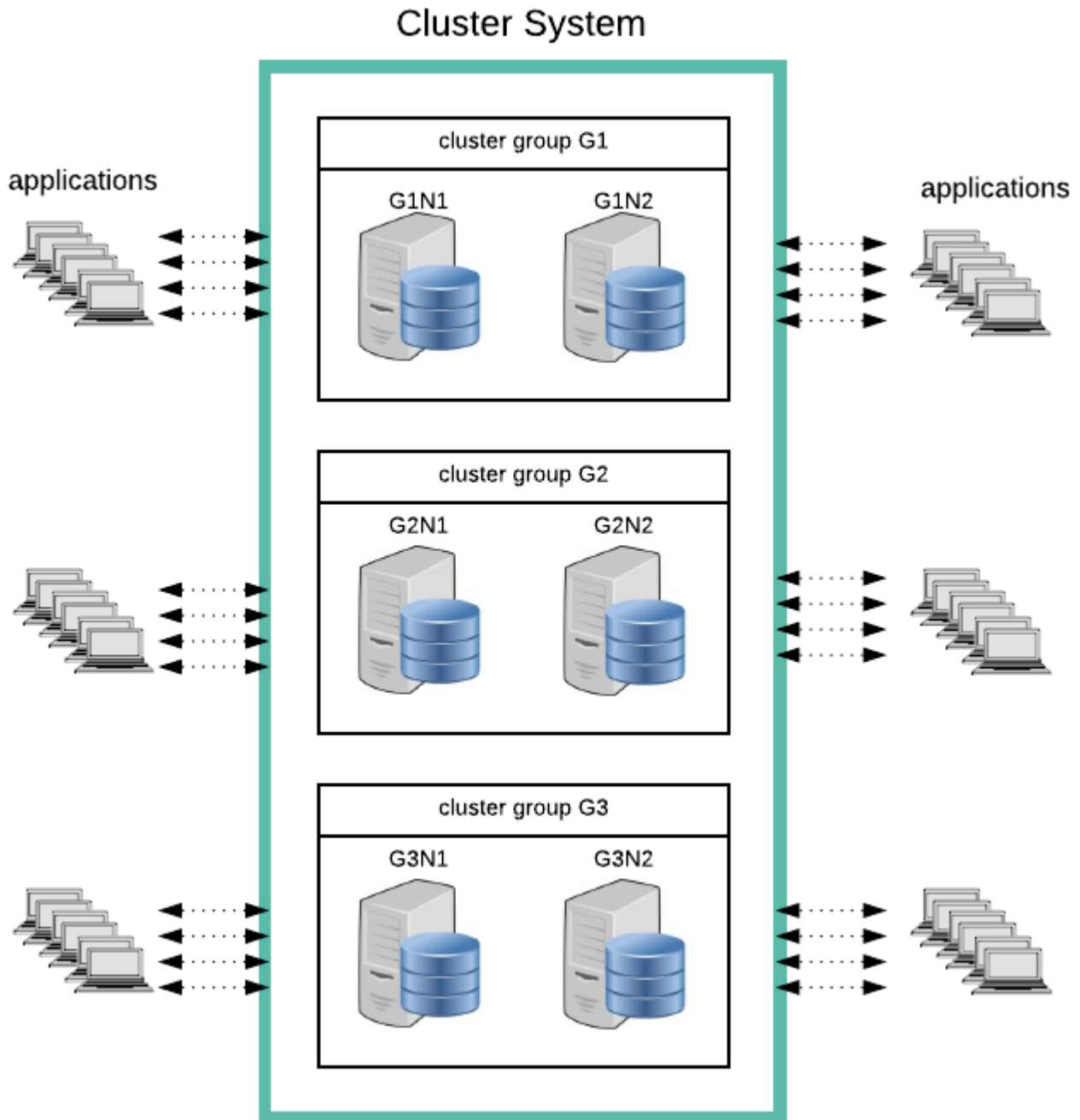
그림 1 3 x 2 cluster system
