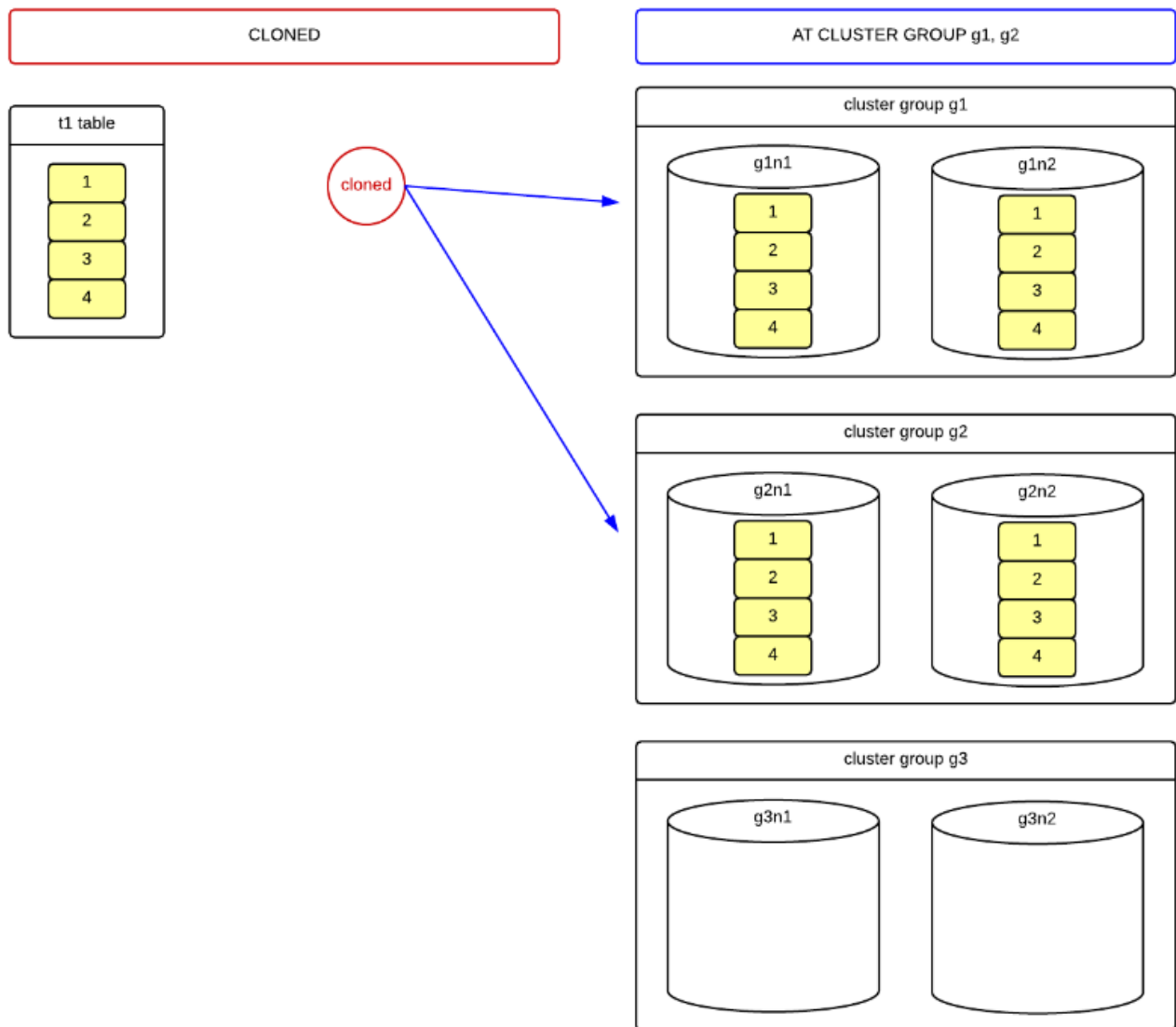
그림 6 Group-specific cloned table
