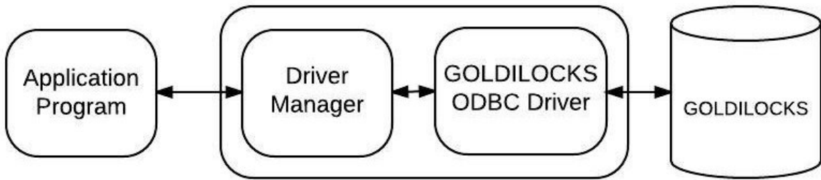
그림 1 드라이버 관리자를 포함하는 GOLDILOCKS ODBC driver
