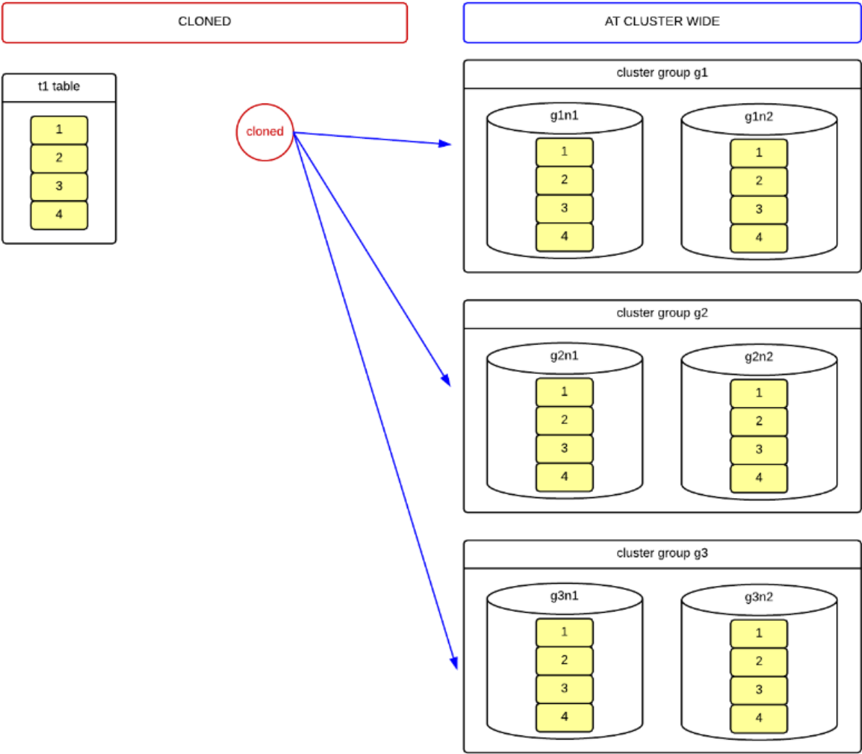
그림 5 Cluster-wide cloned table
