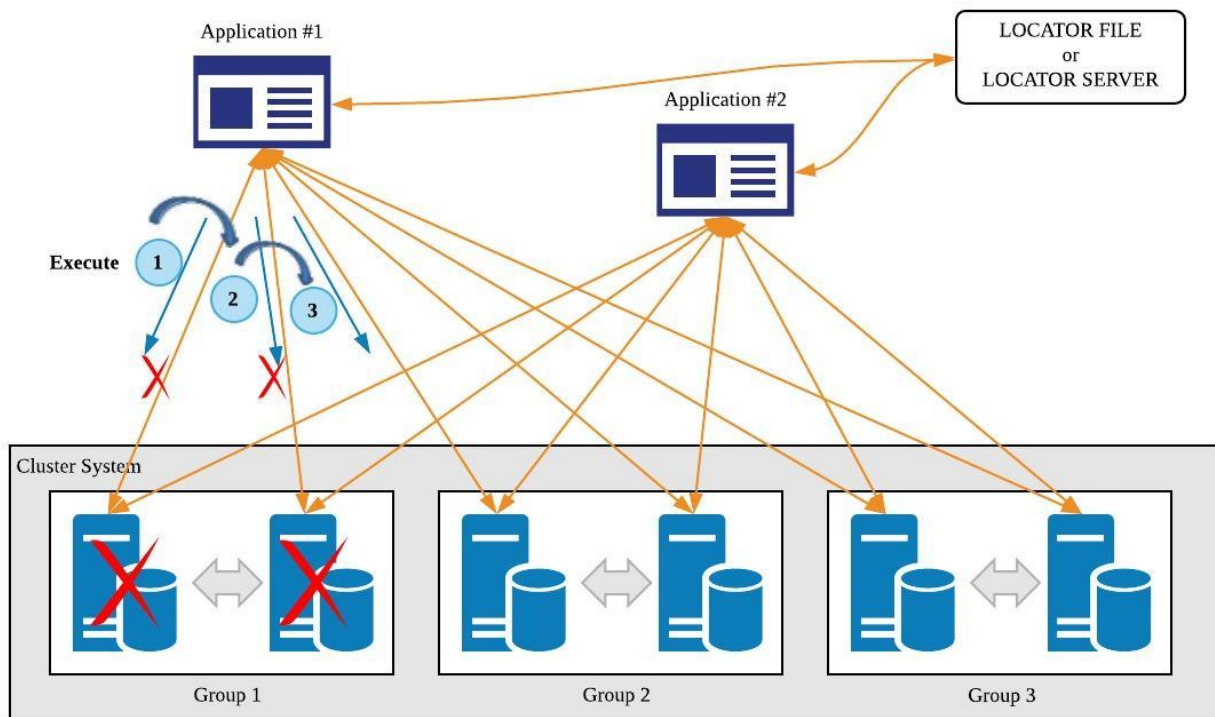
그림 6 GLOBAL CONNECTION HA (high availability)
