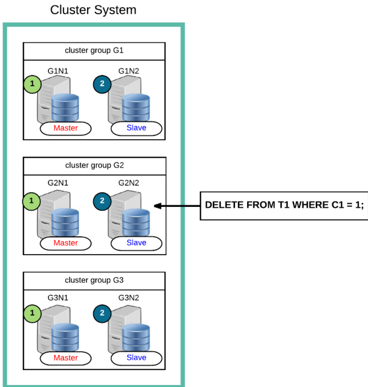
그림 3 Cluster에서의 DML 처리
