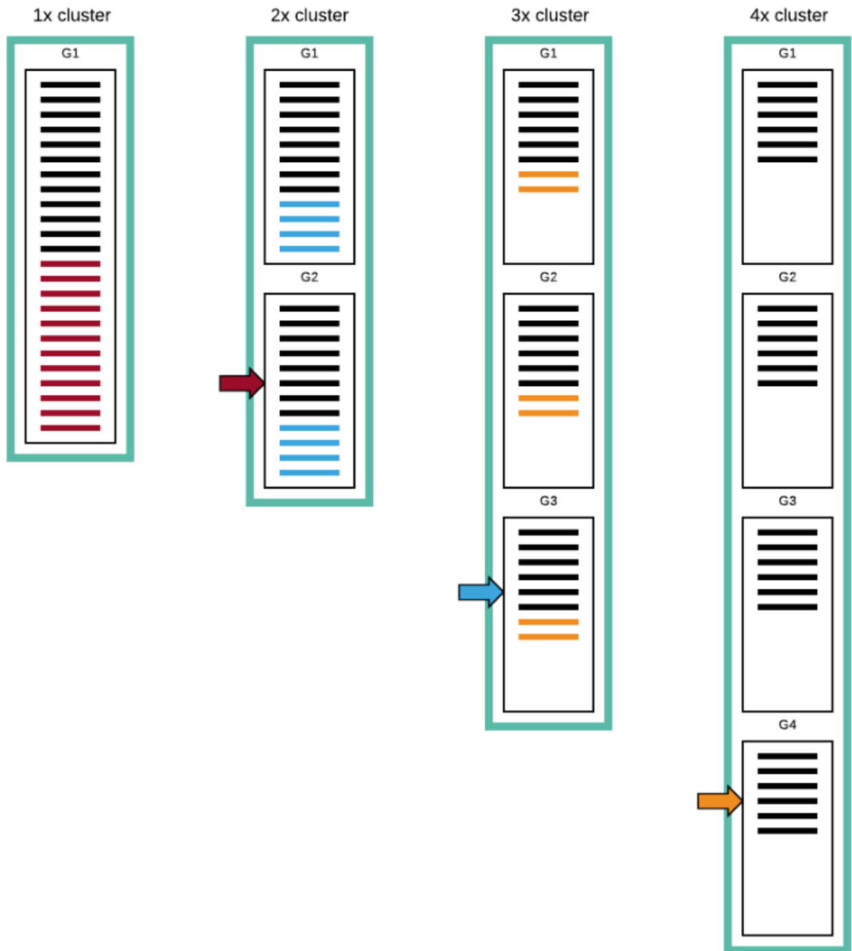
그림 15 Cluster group 증가에 따른 shard 재배치
