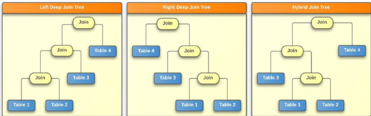
그림 2 Join tree의 종류
