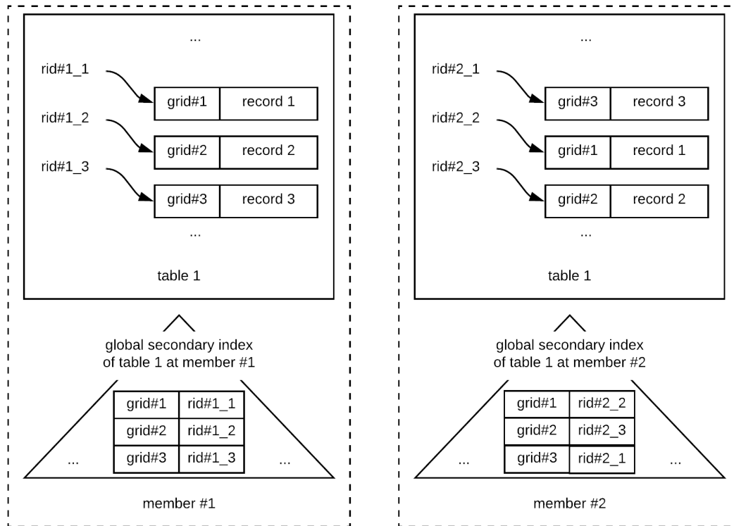
그림 16 Global secondary index 구조
