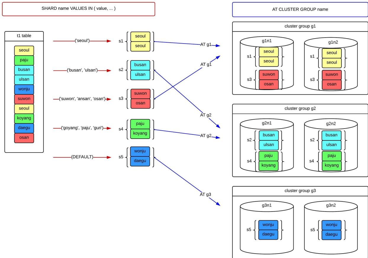
그림 12 Group-specific list-sharded table
