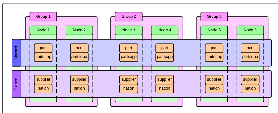
그림 2 3 x 2 cluster 구성과 table
