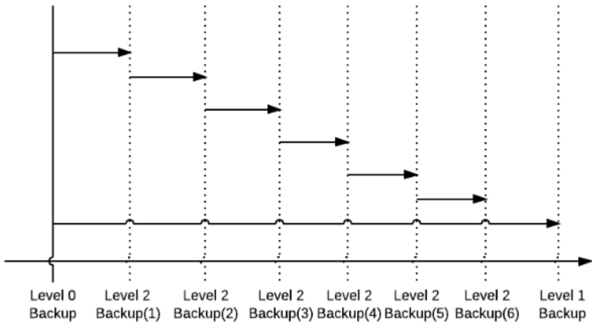
그림 1 Incremental backup
