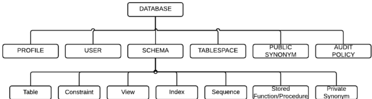
그림 1 SQL objects
