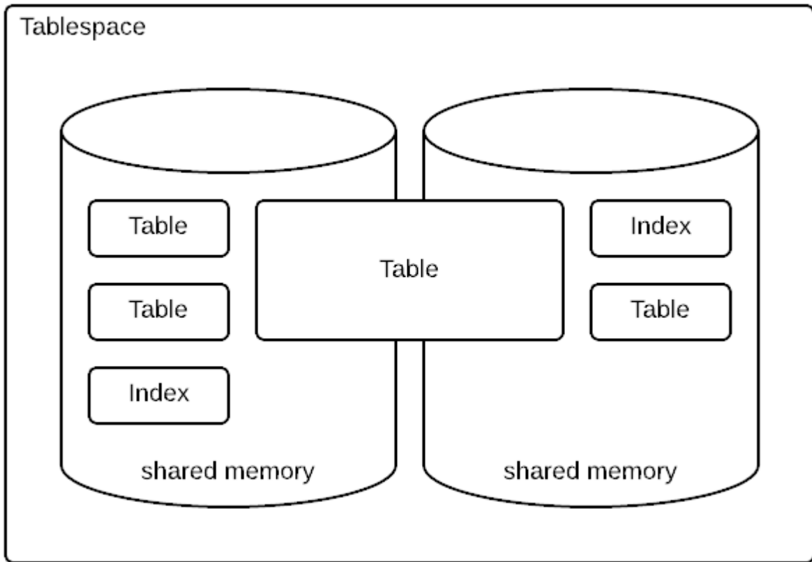
그림 6 Tablespace 개념
