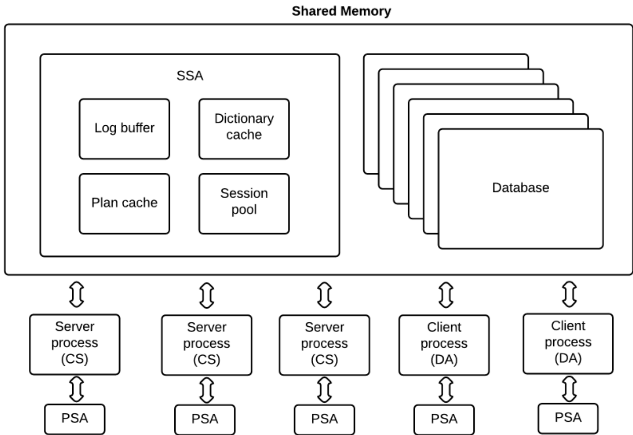
그림 1 Shared Memory
