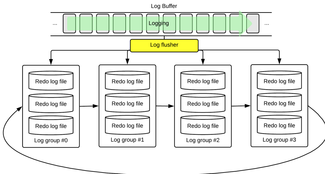
그림 1 GOLDDILOCKS redo log file, 로그 buffer 구조
