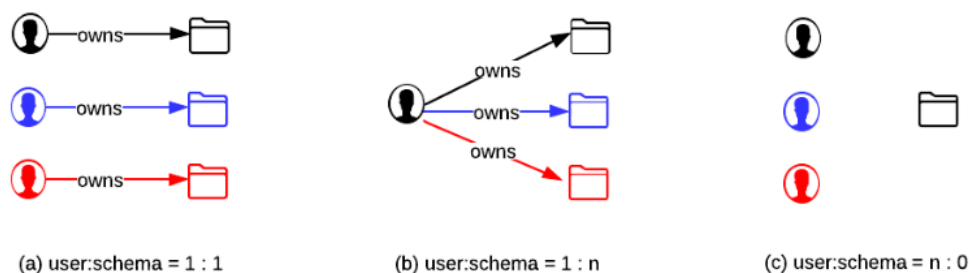
그림 4 User와 schema의 관계
