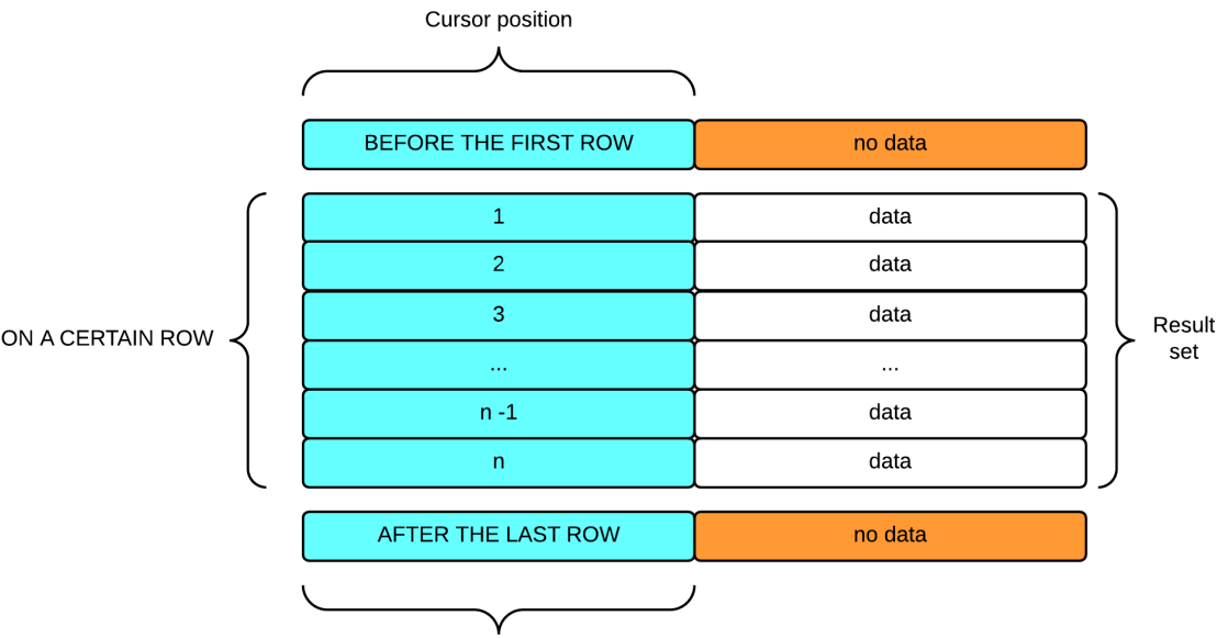
그림 1 커서의 위치 정보
