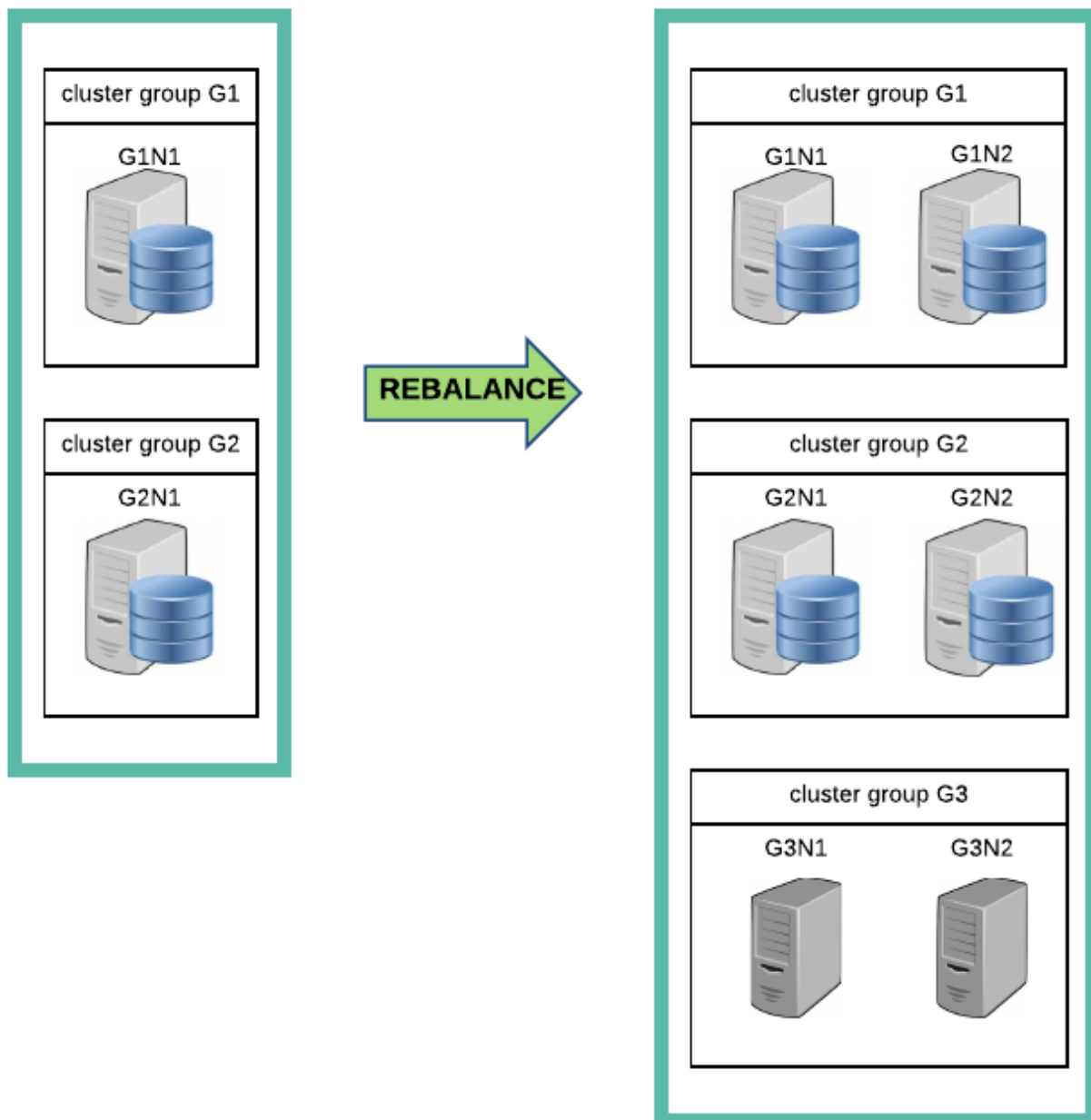
그림 14 AT CLUSTER GROUP으로 정의한 nation 테이블 재배포
