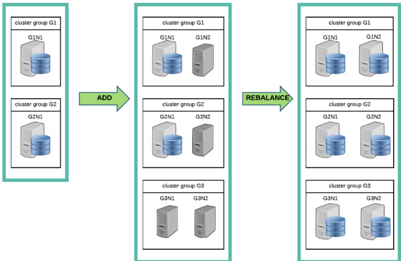
그림 4 Cluster system 확장
