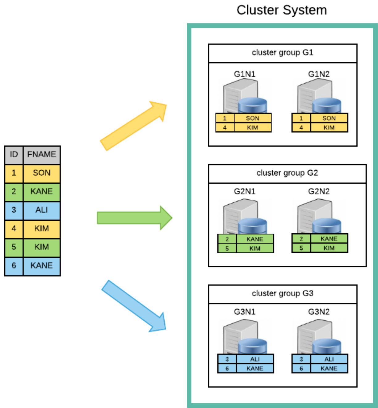
그림 2 Cluster의 분할 및 복제 개념
