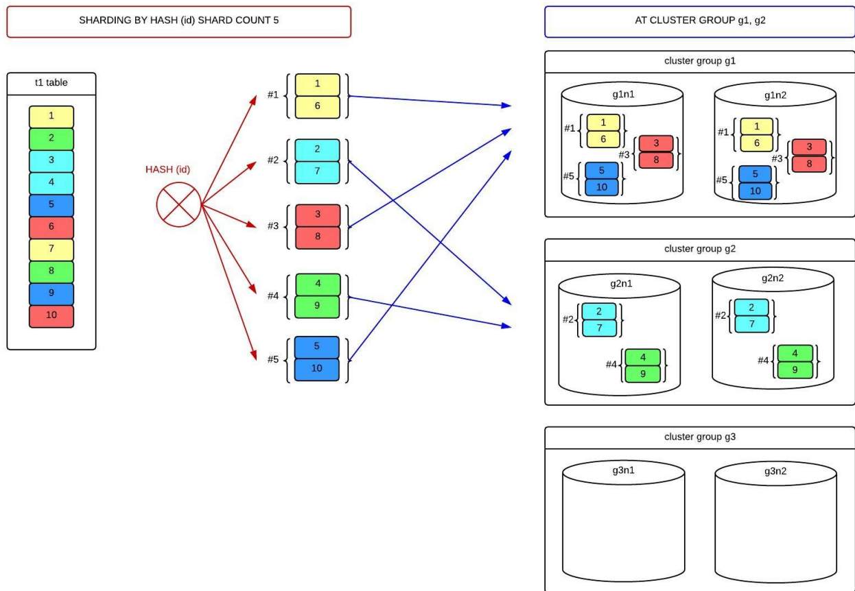
그림 8 Group-specific hash-sharded table
