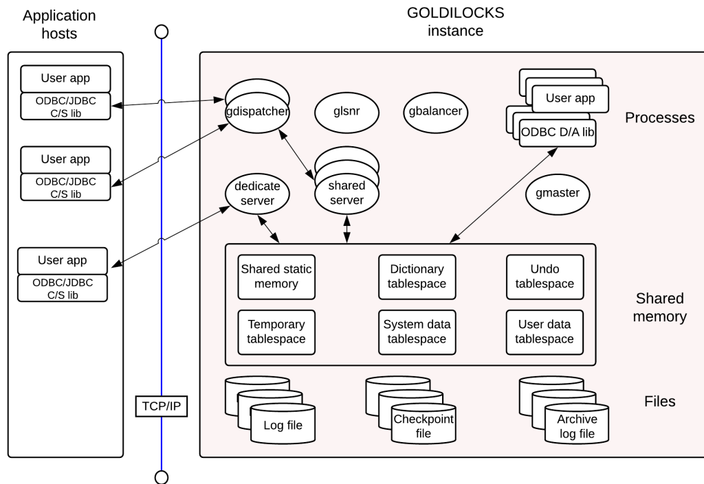
그림 1 GOLDILOCKS architecture
