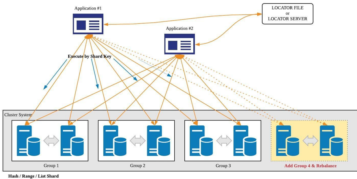
그림 5 GLOBAL CONNECTION
