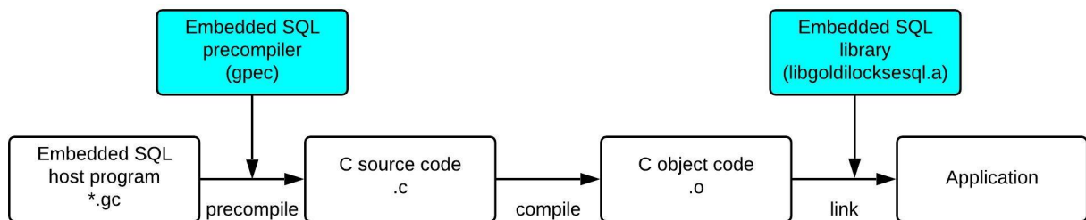
그림 1 Embedded SQL 응용 프로그램 개발
