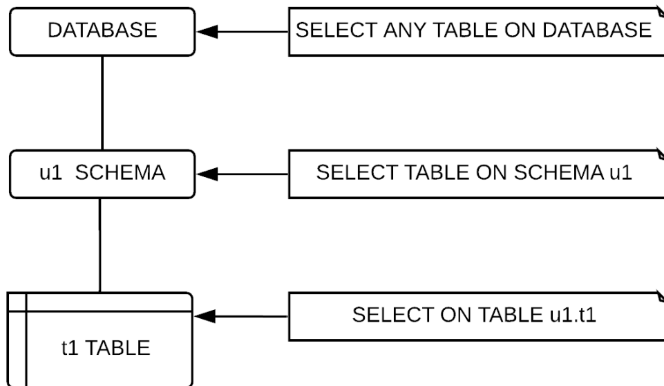
그림 3 SELECT 구문을 수행하기 위한 privilege
