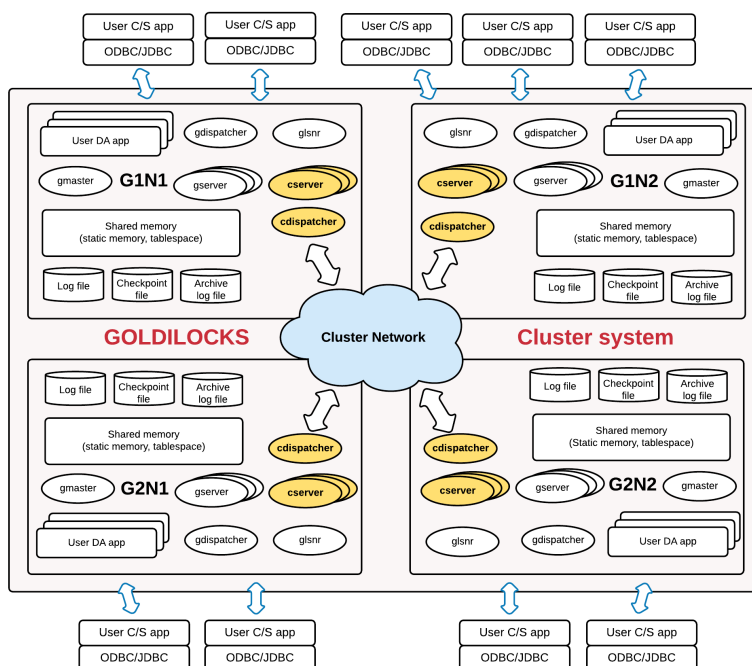
그림 2 GOLDILOCKS cluster system architecture
