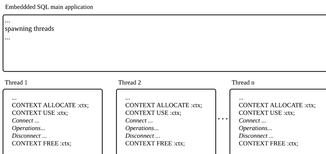
그림 2 D/A 모드에서 각 thread가 각자의 connection을 가지는 경우
