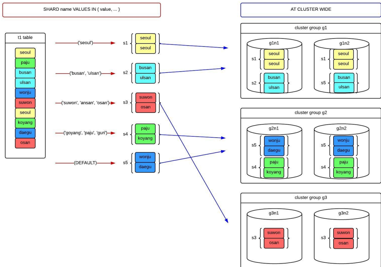
그림 11 Cluster-wide list-sharded table
